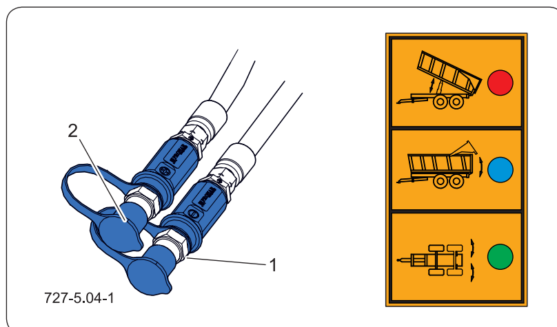
Rysunek 5.14 Przyłącze hydrauliczne
