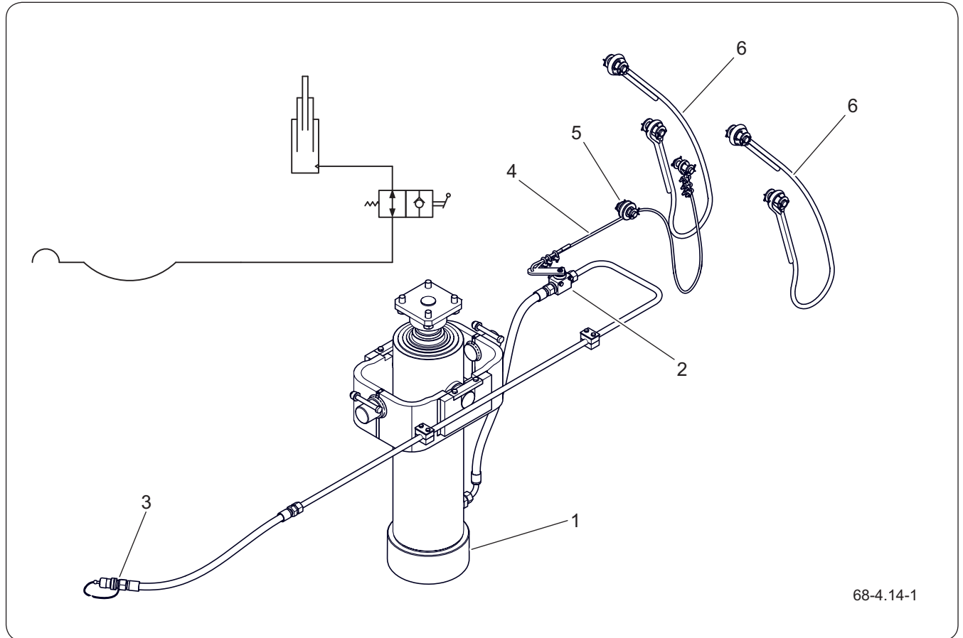
Rysunek 4.5 Budowa i schemat instalacji hydraulicznej wywrotu
