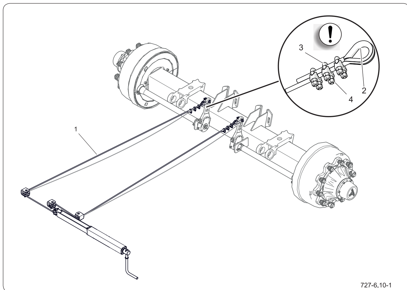
Rysunek 6.20 Wymiana linki hamulca postojowego
