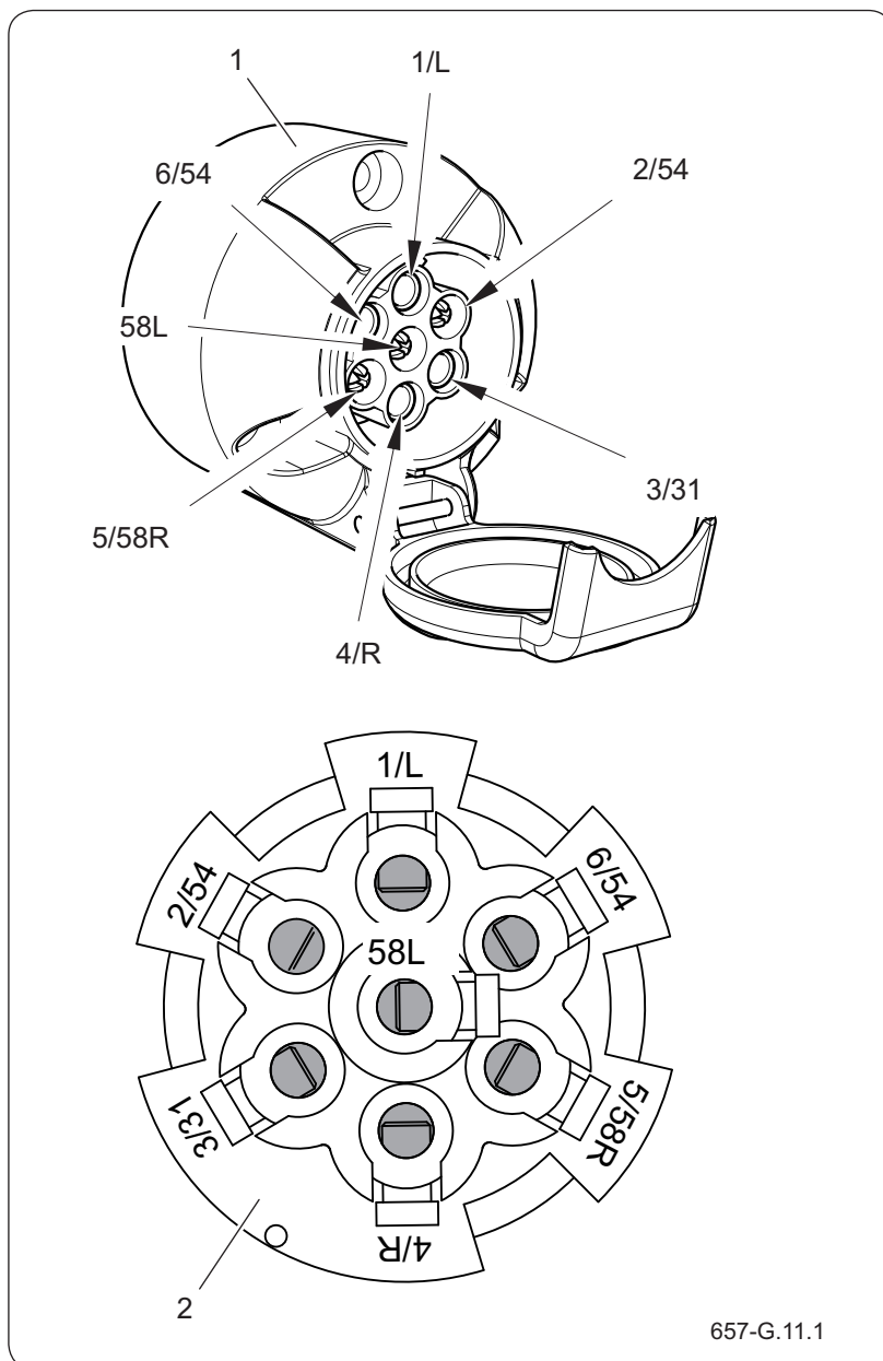
Rysunek 4.11 Gniazdo 7 pin
