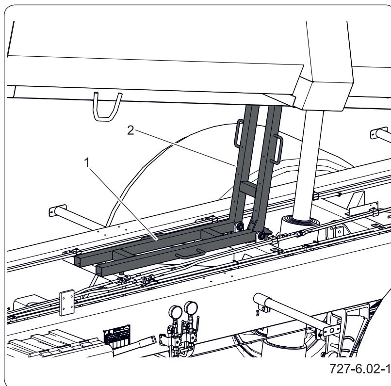
Rysunek 6.3 Podpora skrzyni ładunkowej (1) podpora opuszczona (2) podpora podniesiona
