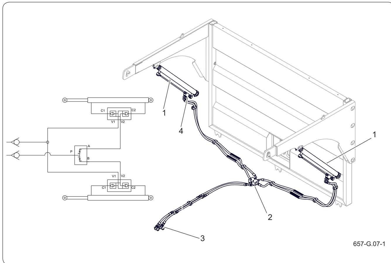
Rysunek 4.6 Budowa i schemat instalacji hydraulicznej klapy tylnej
