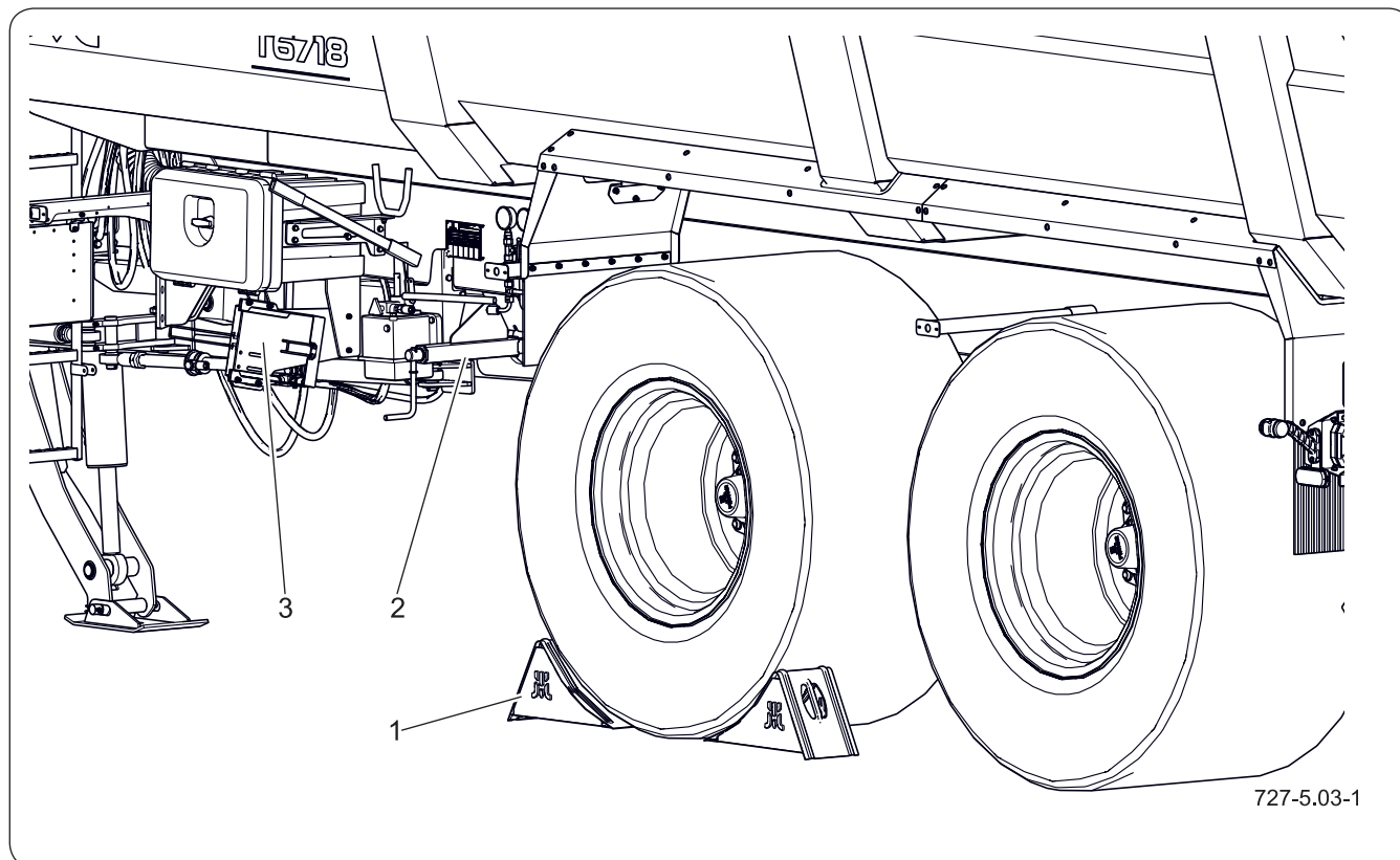
Rysunek 5.11 Hamulec postojowy
