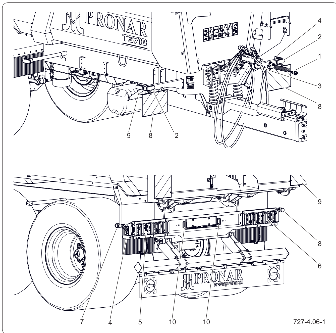
Rysunek 4.10 Rozmieszczenie elementów instalacji elektrycznej oraz elementów odblaskowych - belka oświetleniowa pełna.
