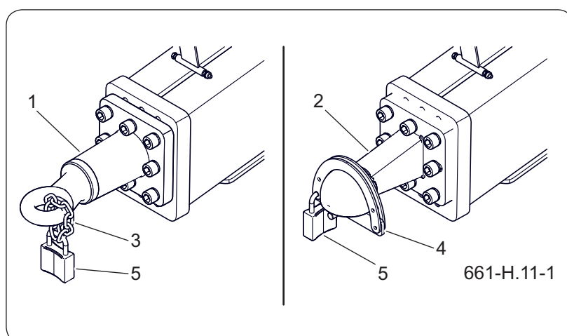
Rysunek 5.12 Zabezpieczenie ciągną dyszla
