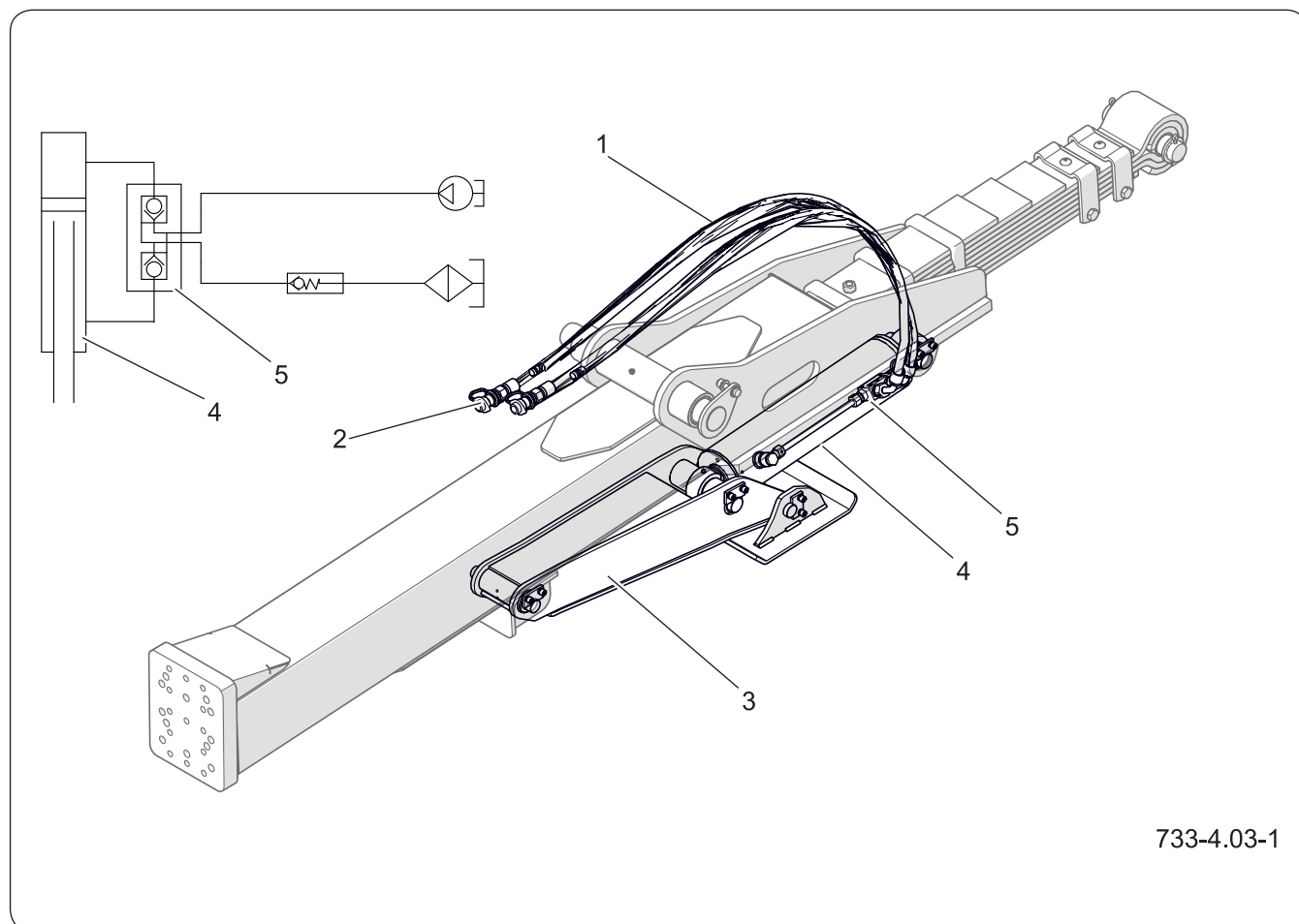
Rysunek 4.7 Budowa i schemat instalacji hydraulicznej podpory nożycowej
