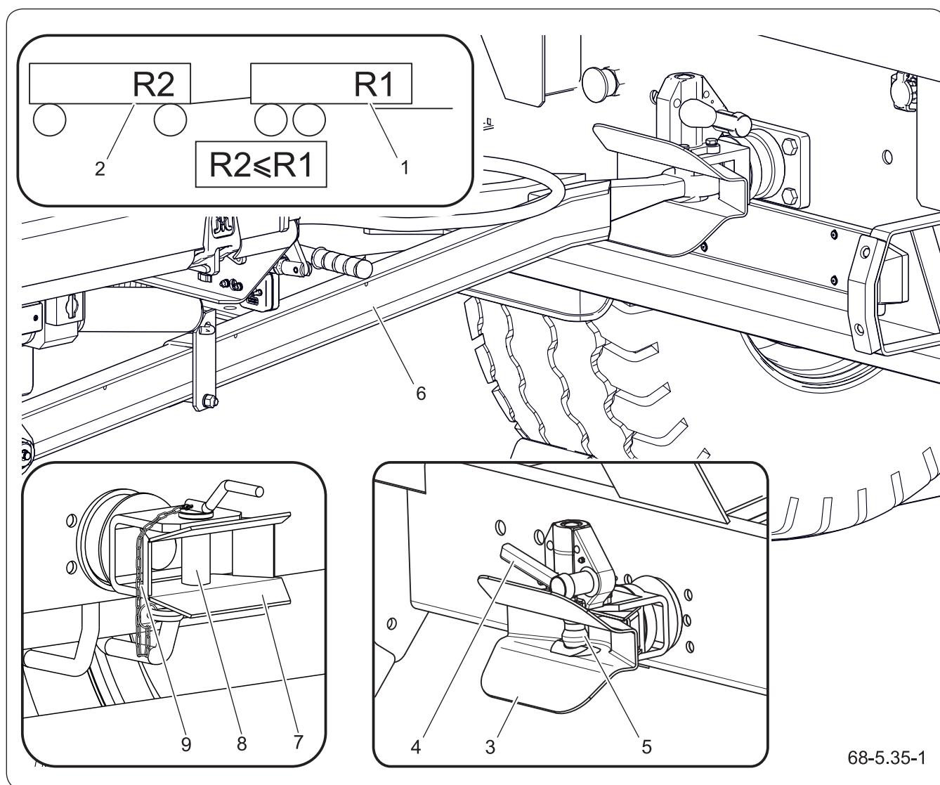
Rysunek 5.22 Agregowanie drugiej przyczepy
