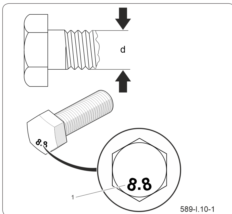
Rysunek 6.22 Śruba z gwintem metrycznym (1) klasa wytrzymałości (d) średnica gwintu
