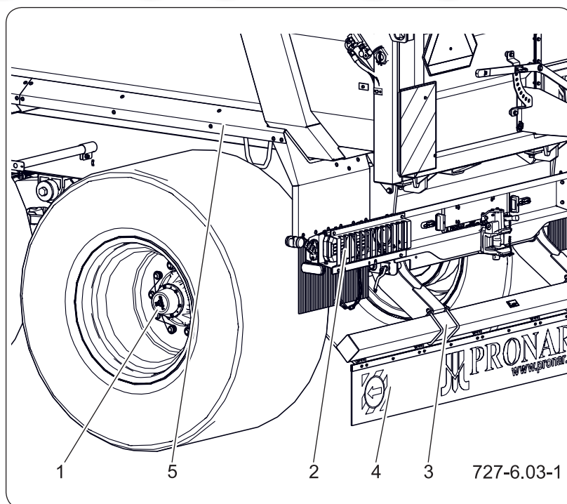
Rysunek 6.5 Osłony przyczepy
