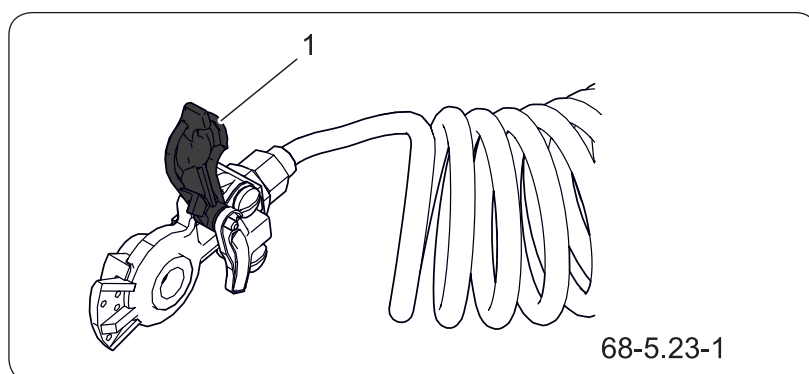
Rysunek 5.17 Instalacja hamulcowa jedнопrzewodowa (1) wtyk czarny
