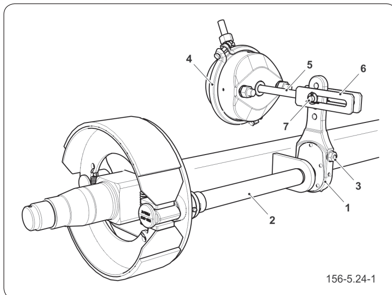
Rysunek 6.17 Hamulec pneumatyczny osi jezdnej
