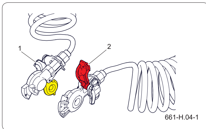
Rysunek 5.13 Przewody instalacji hamulcowej pneumatycznej
