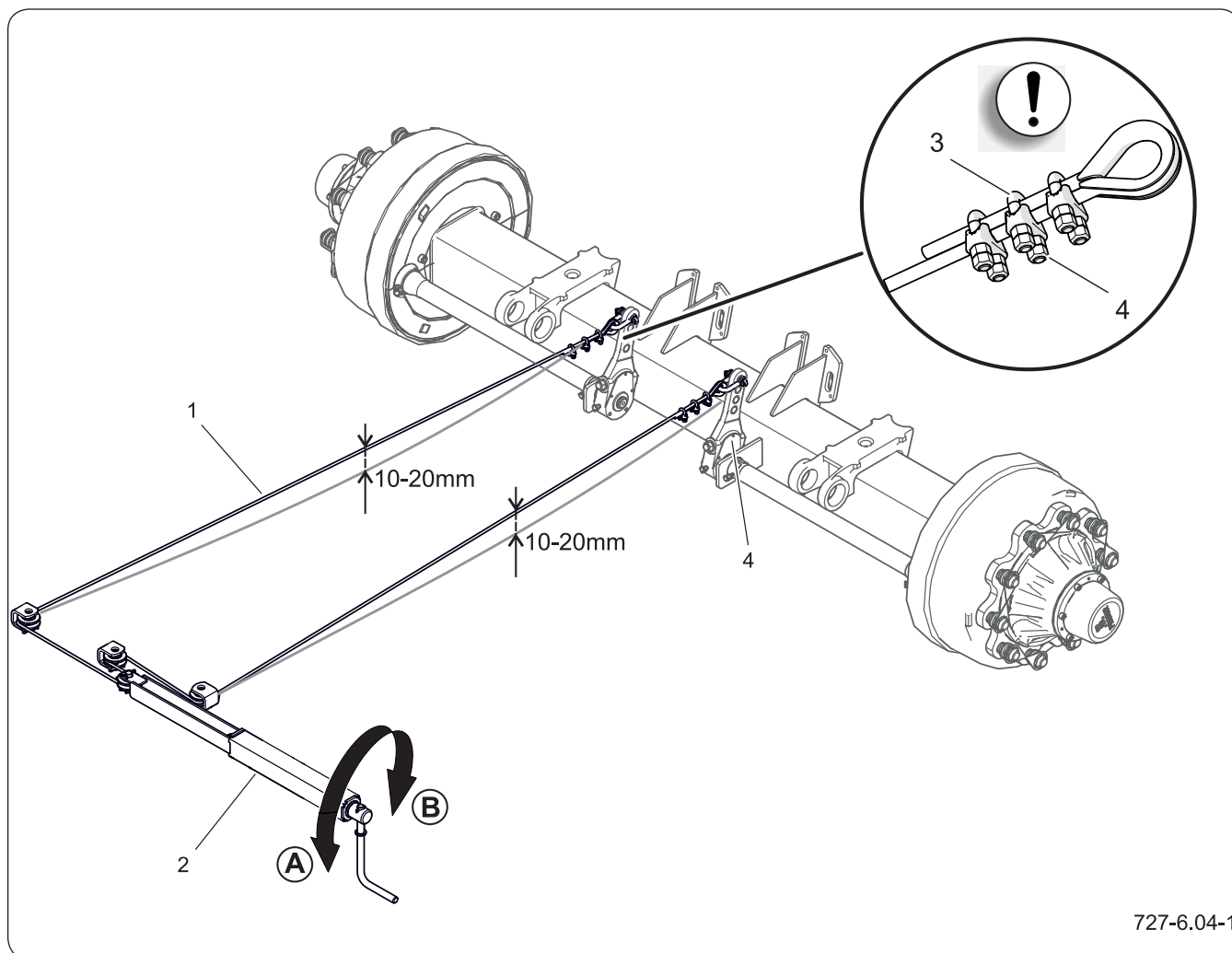
Rysunek 6.19 Kontrola napięcia linki
