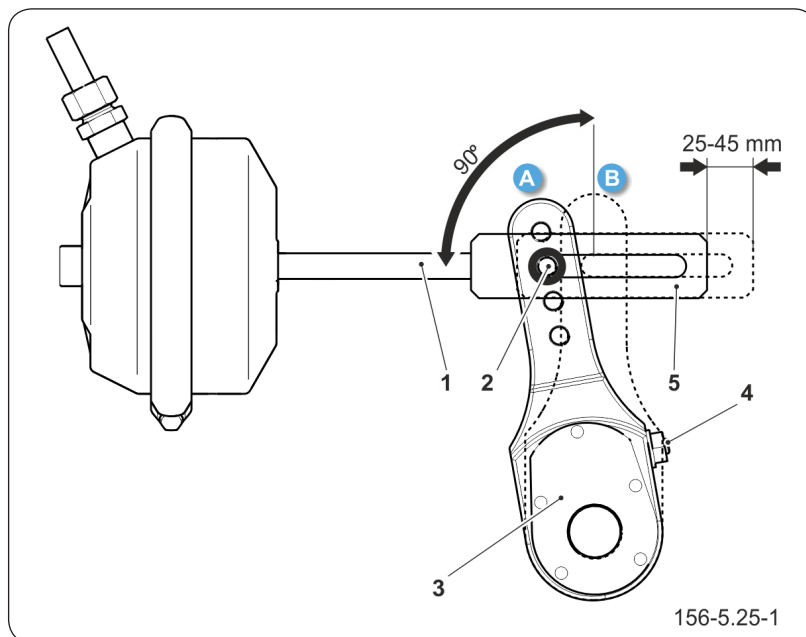
Rysunek 6.18 Regulacja hamulca
