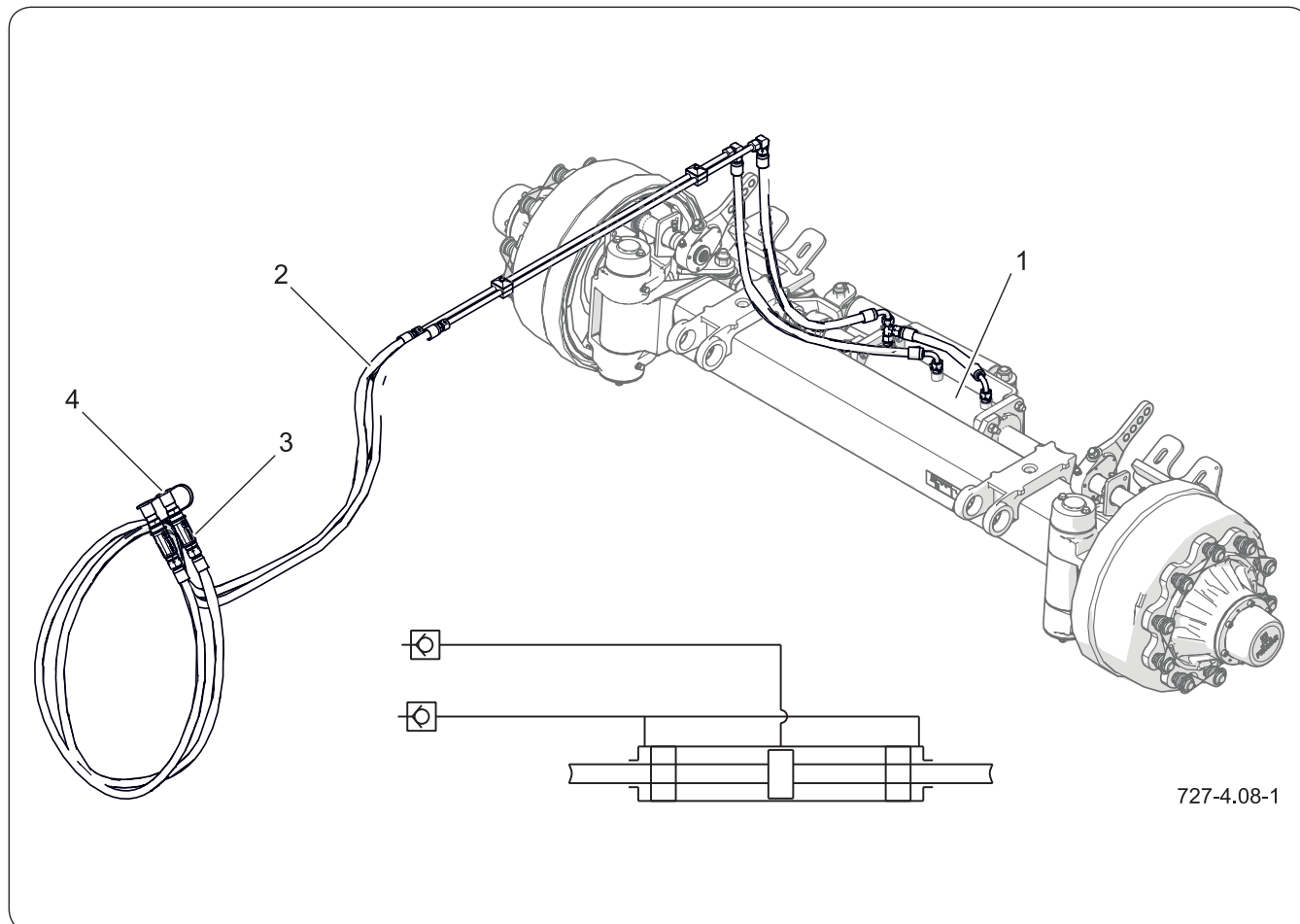
Rysunek 4.8 Budowa i schemat instalacji hydraulicznej blokady skrętu
