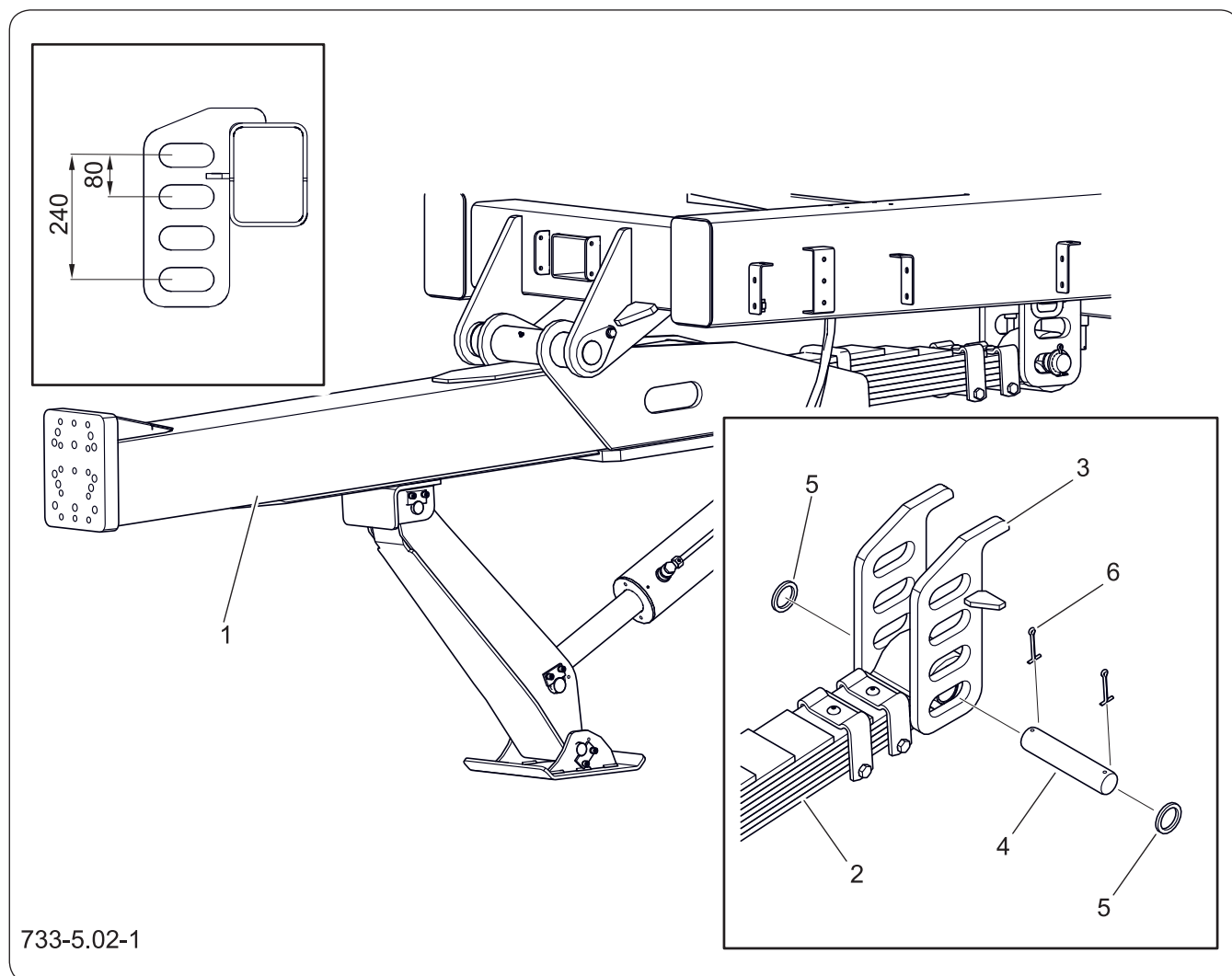
Rysunek 6.1 Amortyzacja mechaniczna dyszla
