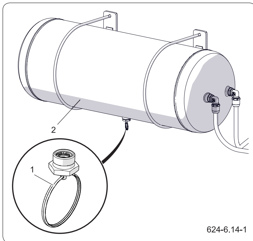
Rysunek 6.7 Zbiornik powietrza
