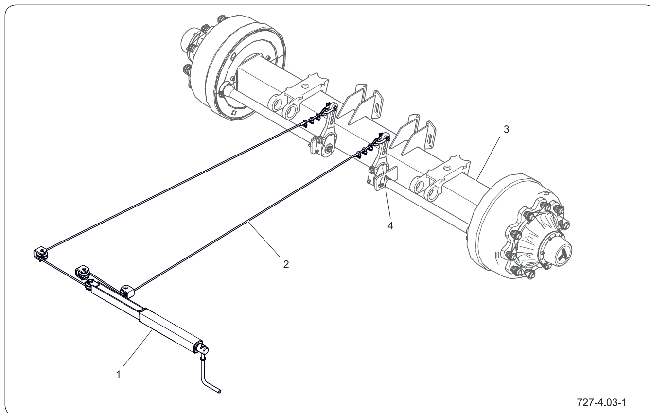
Rysunek 4.4 Budowa hamulca postojowego
