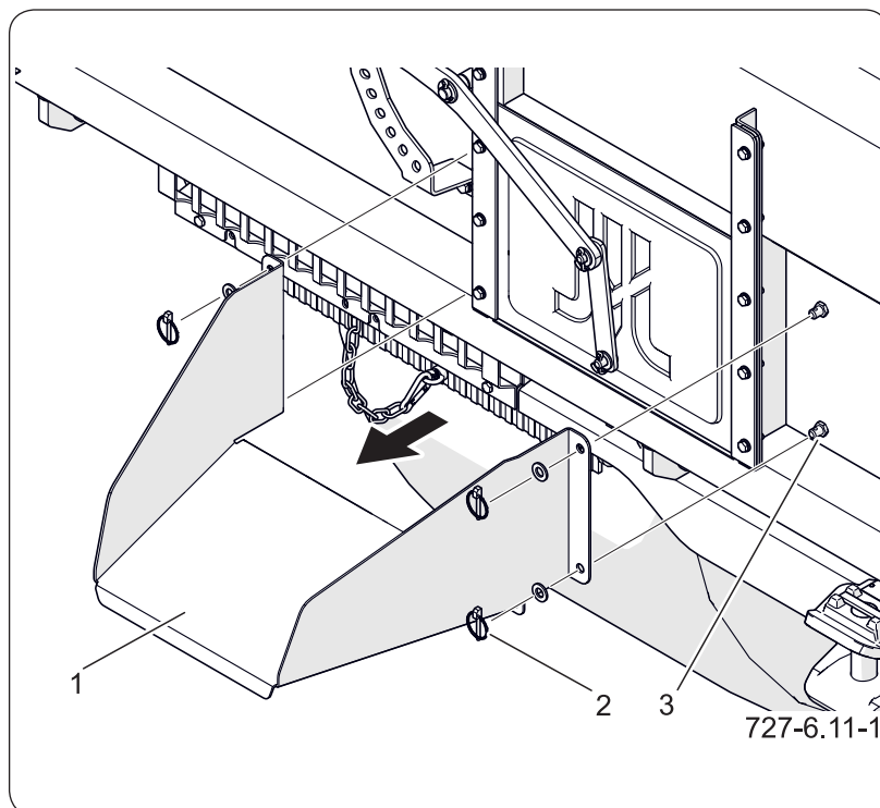
Rysunek 6.24 Rynna zsypowa
