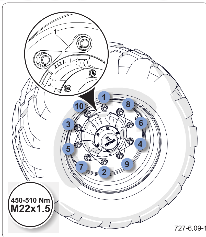
Rysunek 6.13 Kolejność dokręcania nakrętek (1) wskaźnik dokręcenia nakrętki
