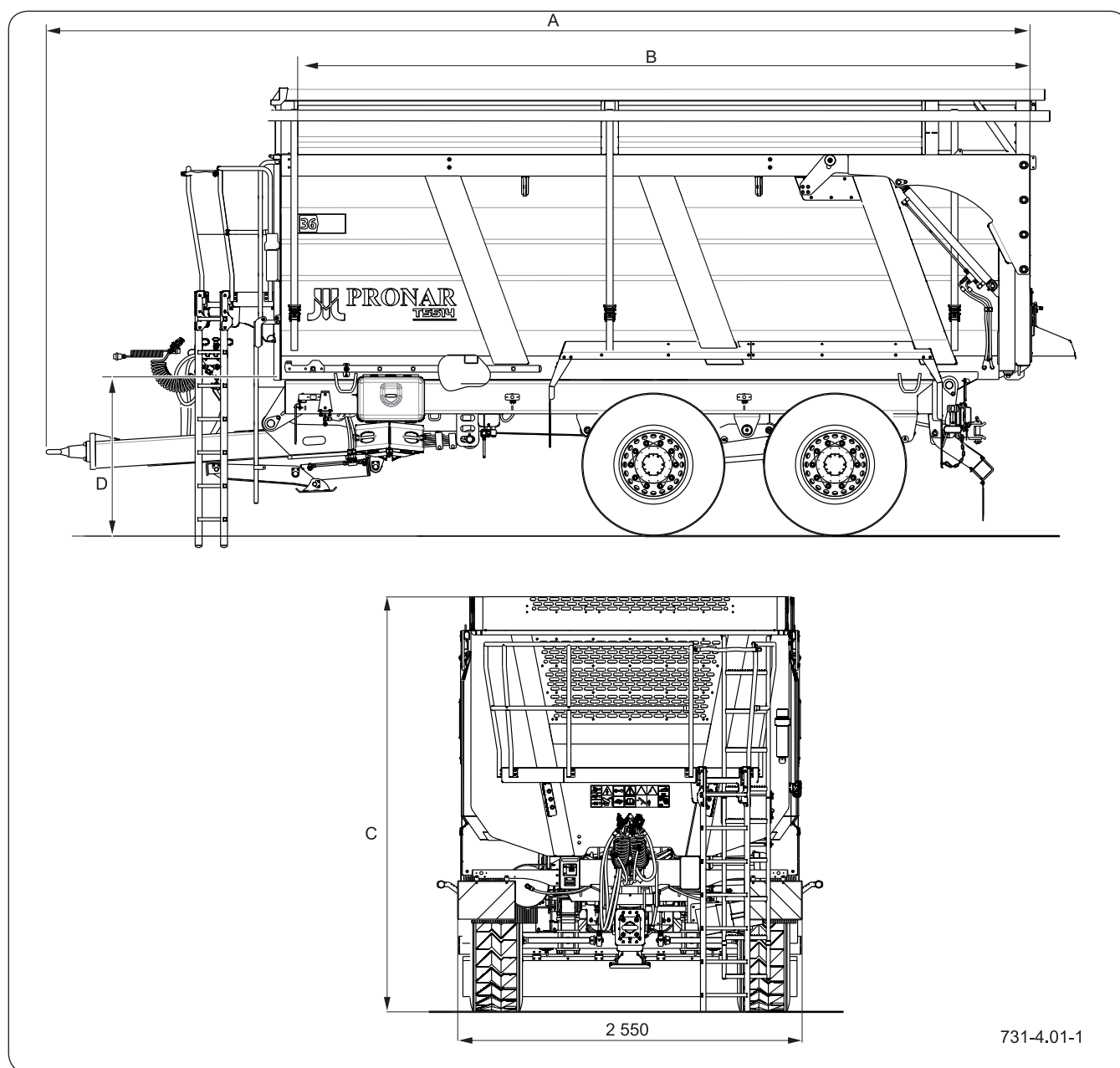
Rysunek 4.1 Podstawowe wymiary przyczepy
