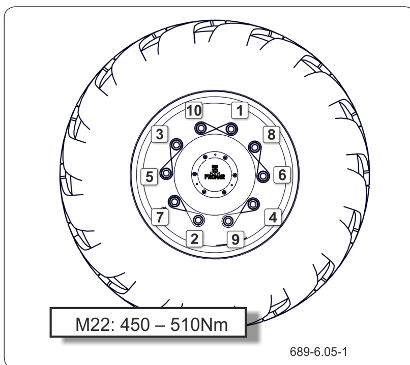
Rysunek 6.12 Kolejność dokręcania nakrętek
