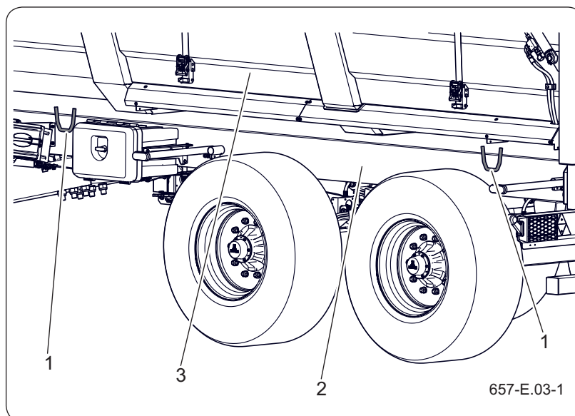
Rysunek 2.8 Punkty mocowania
