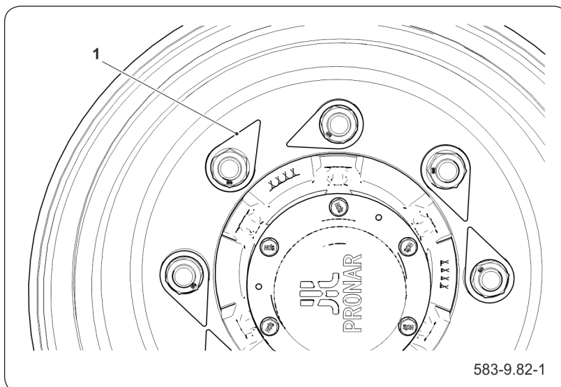
Rysunek 6.14 Wskaźniki dokręcenia
